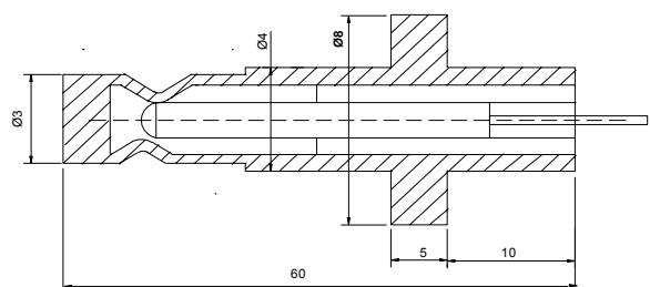
Messaufnehmer: Messzelle und Gehäuse
